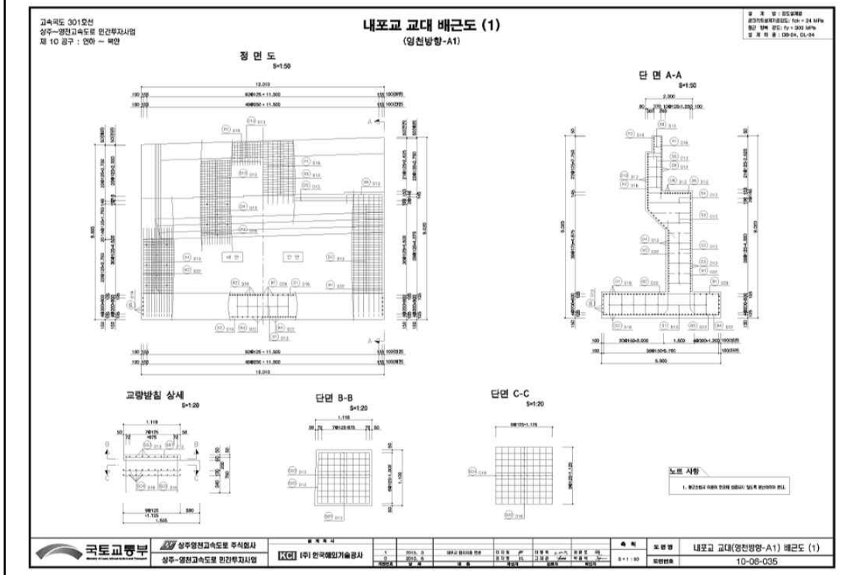
【그림 30.1.13】 교대 배근도
